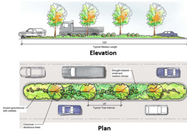
Median Enlargement
